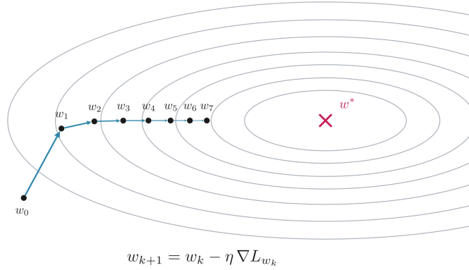
Рис. 8: Траектория градиентного спуска.
