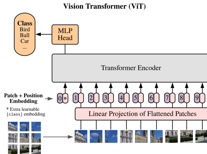
Рис. 22: Архитектура ViT. Взято из оригинальной статьи “An Image is Worth 16x16 Words”.
