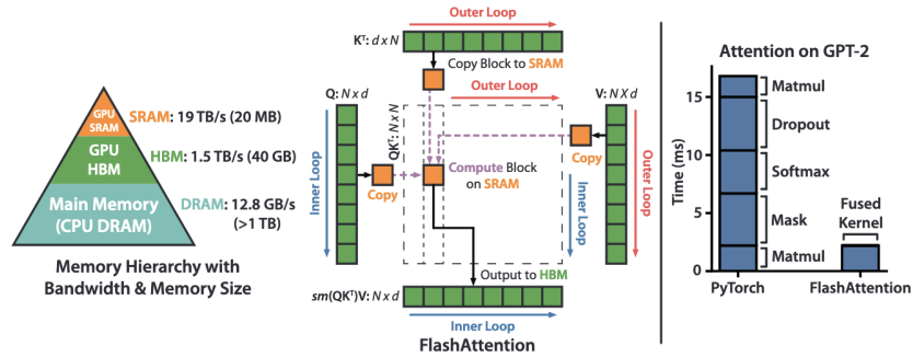
Рис. 28: Схема Flash Attention.
