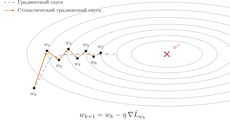
Рис. 9: Траектория стохастического градиентного спуска.
