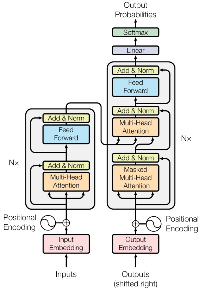
Рис. 21: Архитектура трансформера кодировщика-декодировщика, взято из оригинальной статьи "Attention is all you need".
