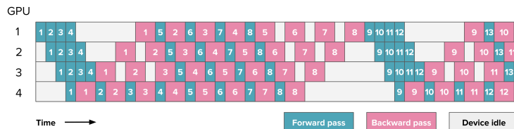
Рис. 48: 1F1B. Взято из Ultra-Scale Playbook.
