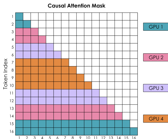
Рис. 44: Распределяем токены так, чтобы выровнять нагрузку на ранги. Взято из Ultra-Scale Playbook.
