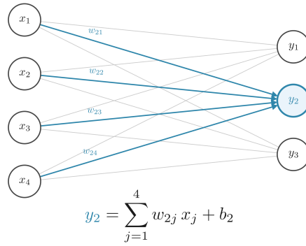
Рис. 1: Схема полносвязного слоя.
